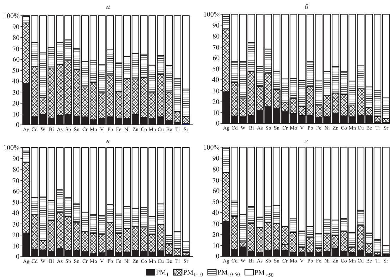
Рис. 3. Доля ТМ в гранулометрических фракциях дорожной пыли: а — малые дороги, б — средние дороги, в — крупные дороги, з — МКАД
